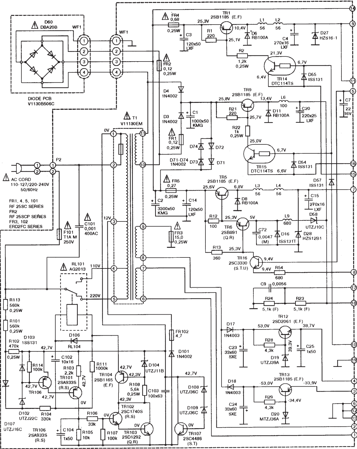
Принципиальная схема трансформаторного блока источника питания видеомагнитофона VS-G40EM
